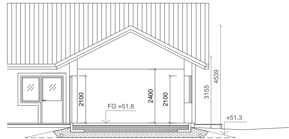
SEKTION
